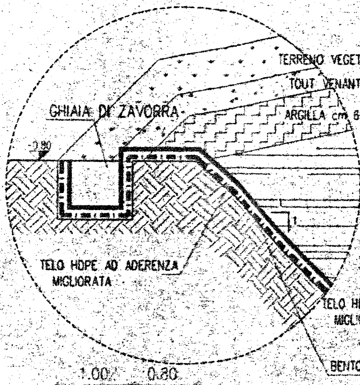
DETTAGLIO A SCALA 1:50
