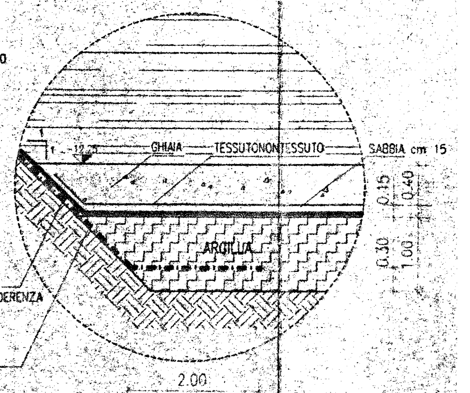
DETTAGLIO B SCALA 1:50
